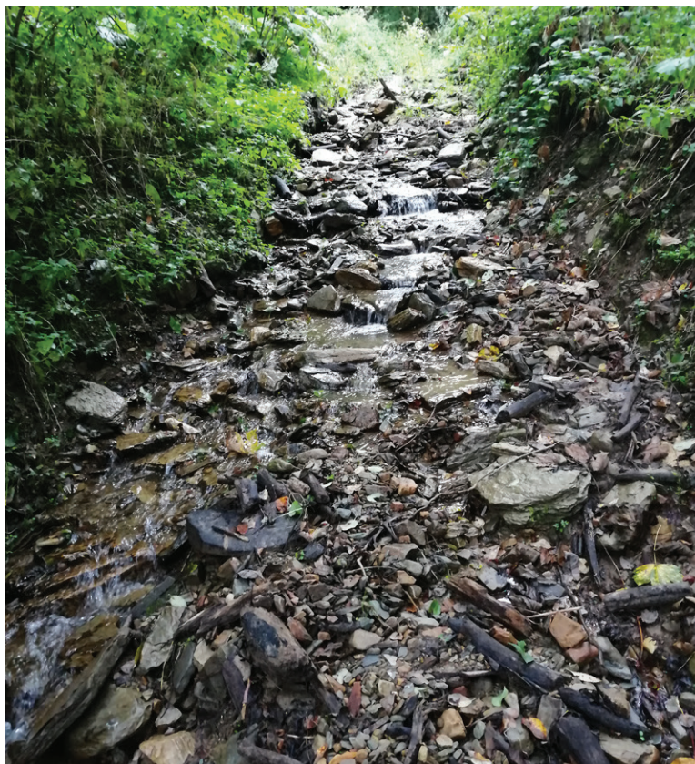
Slika 7. Ekstremna uticaja traktorskog puta na odvodnju površinskih voda (kategorija V) / Figure 7. Extreme impact of skid roads on the drainage of surface water (category V)
